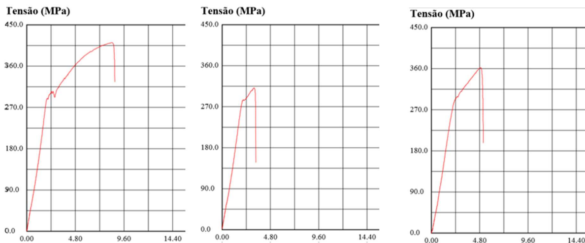
Figura 6 - Gráfico de tensão do Eletrodo Revestido
