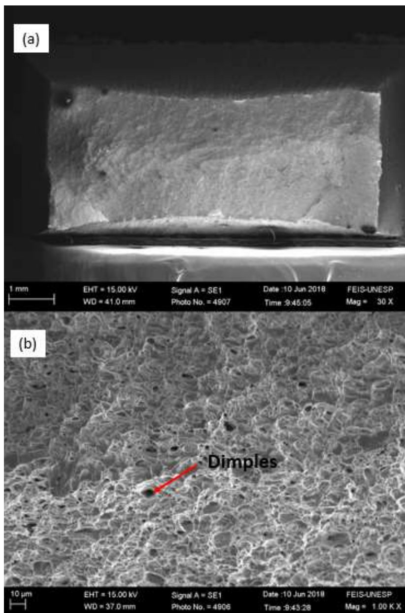
Figura 9 - Microscopia do material sem solda
