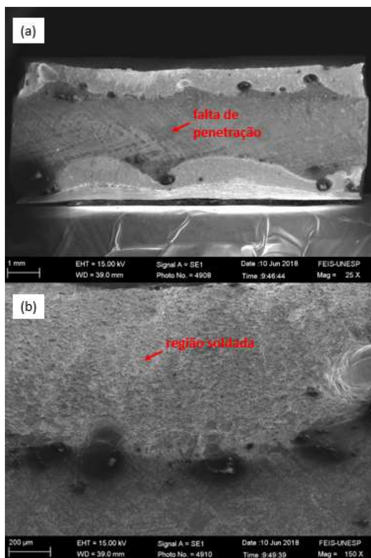
Figura 11 – Microscopia da soldagem MAG
