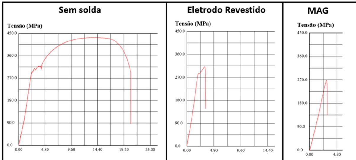
Figura 8 – Comparação dos gráficos em cada processo.
