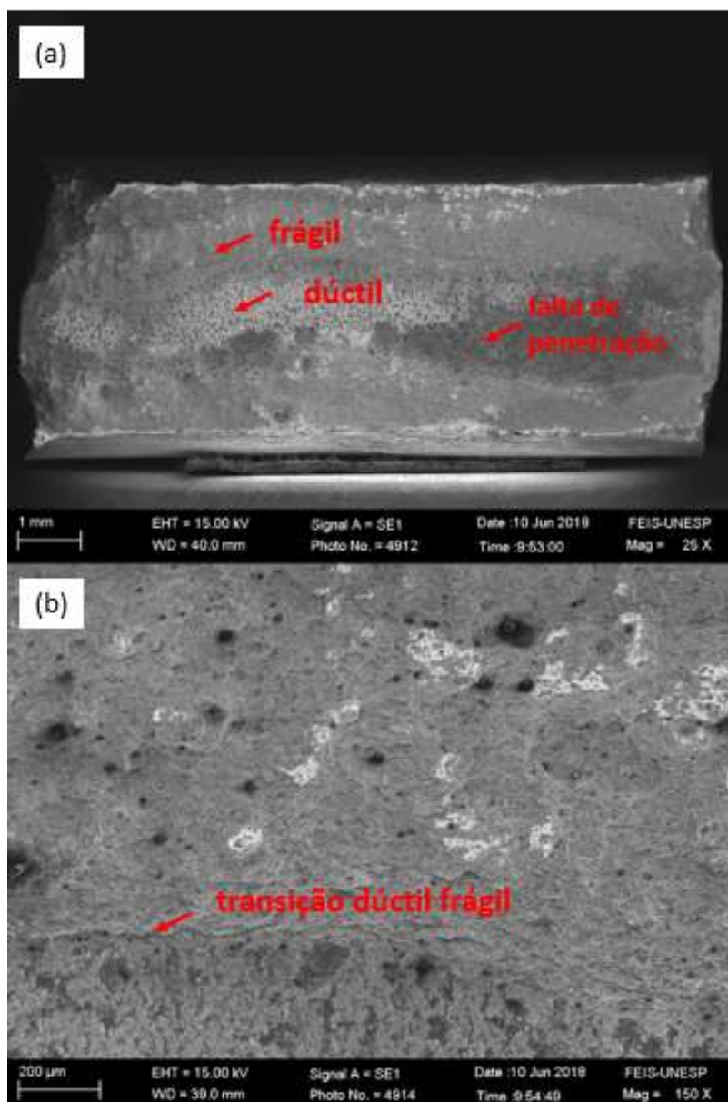
Figura 10 – Microscopia da soldagem por Eletrodo Revestido
