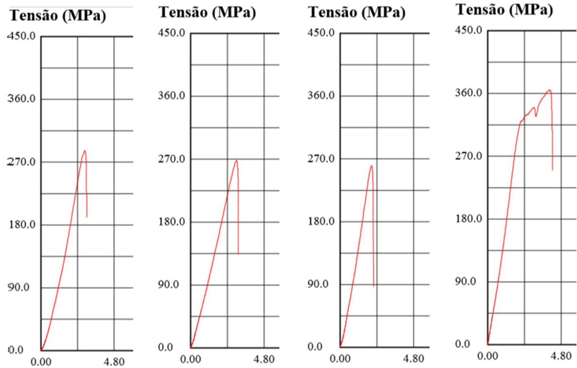
Figura 7 - Gráfico de tensão por MAG
