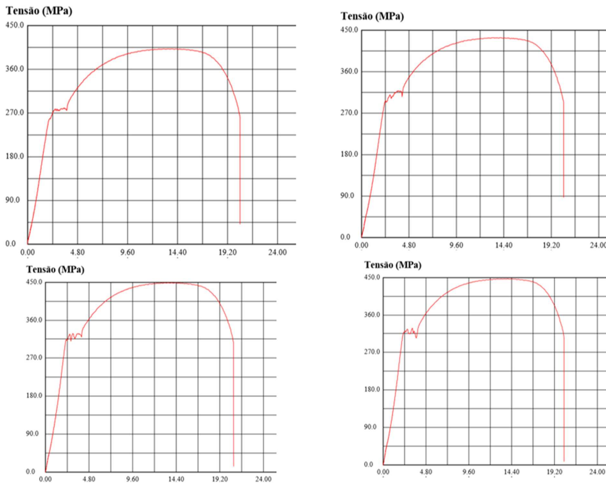
Figura 5 - Gráfico de tensão do material Sem Solda
