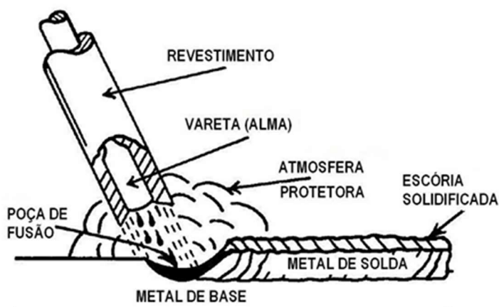
Figura 1 - Soldagem a arco elétrico com eletrodo revestido
